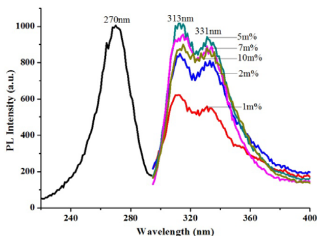
Fig. 6 PL spectra of \text{K}_2\text{CaSr}(\text{SO}_4)_3:\text{xCe}^{3+} 270nm excitation. ( \lambda_{\text{emi}}=313\text{nm} )
